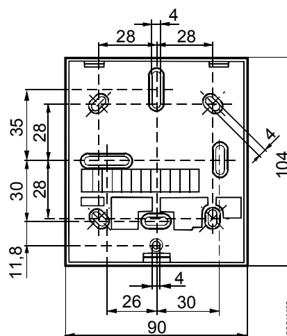
Podstawa montażowa
